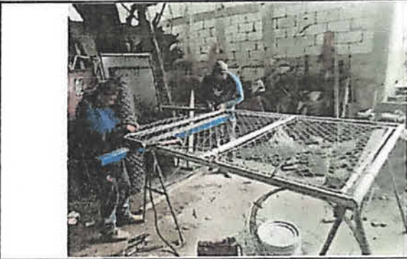
Foto 4: Fabricación del portón de malla de dos hojas abatibles en ambos sentidos con sus pasadores y mecanismo para la colocación de candado en la entrada principal.
